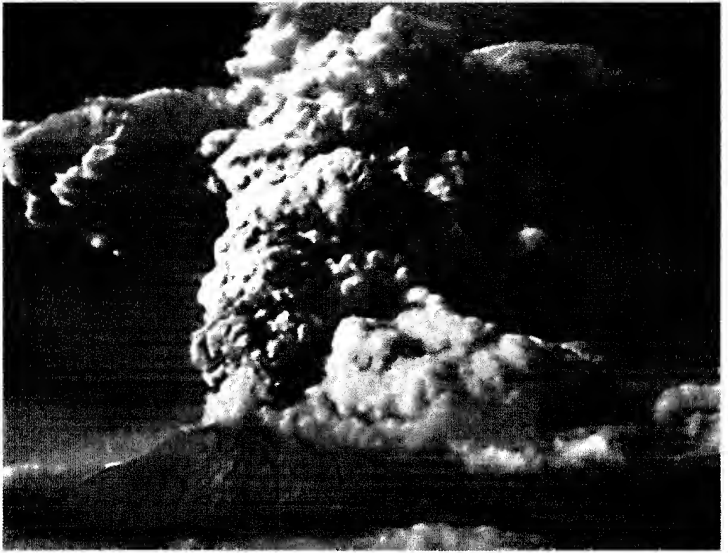
سحب بركانية ضخمة تتصاعد من بركان سانت هيلين بولاية واشنطن سيائل
